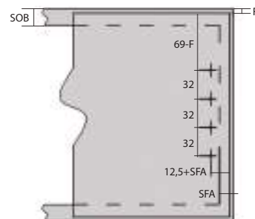
-SFA grosor del módulo-descuento de puerta -F Descuento puerta
