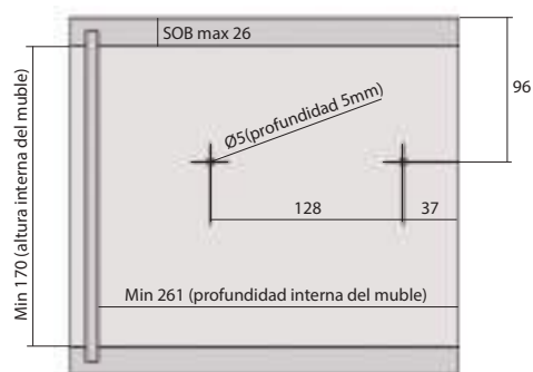
SOB Grosor del panel superior
