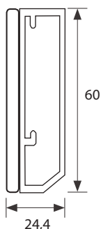
"L" Bastidor
