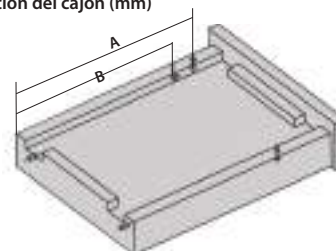
Preparación del cajón (mm)
