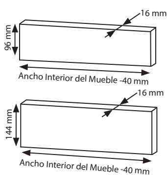
Trasera de Cajón
