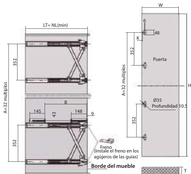
Medidas de instalación para 2 mecanismos
