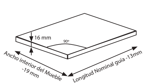
Fondo Cajón
