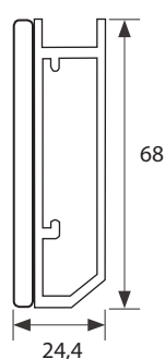
"L" Sin Tirador
