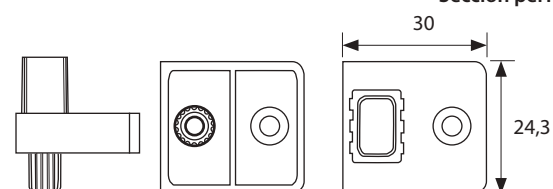
Sección perfil
