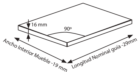
Fondo Cajón
