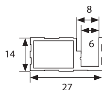
sección perfil
