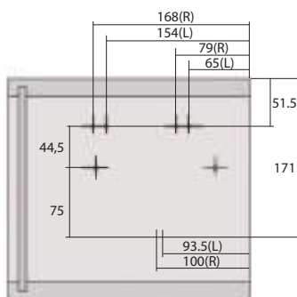
Fijación de posiciones
