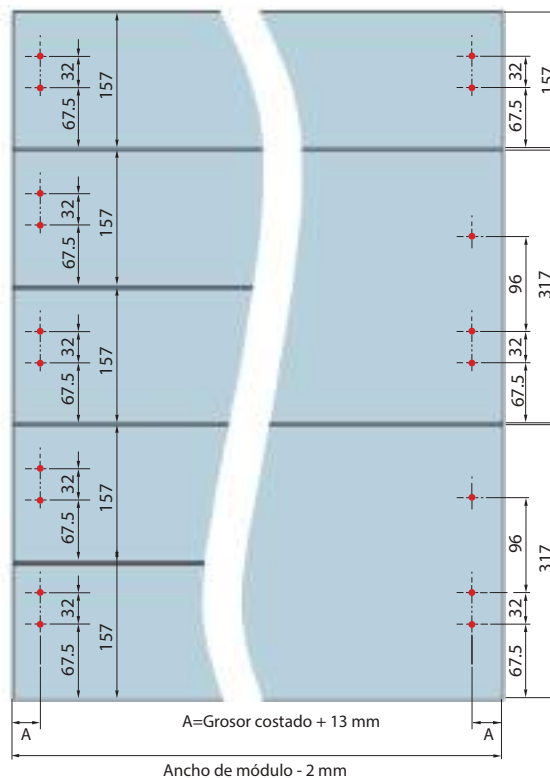
Trasera de Cajón
