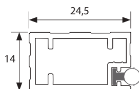
Sección perfil
