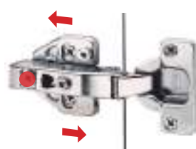
Ajuste profundidad +3 mm/-2 mm
