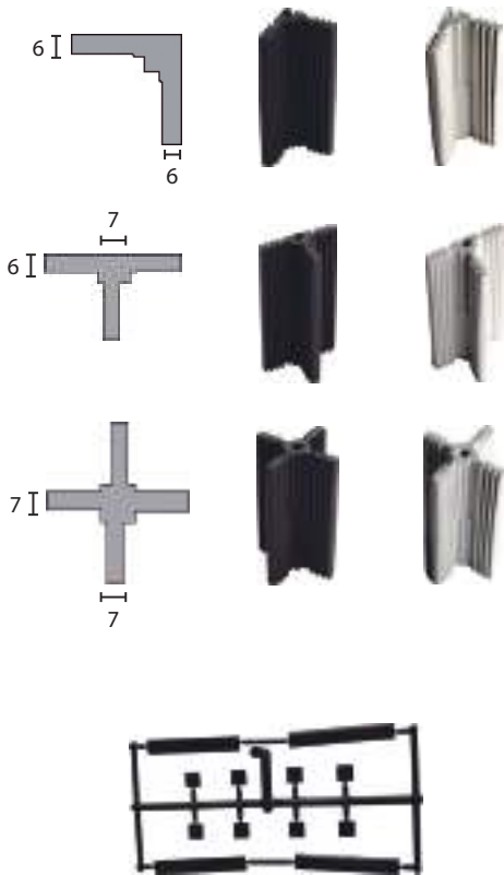
Kit de tapas
