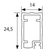
Sección perfil
