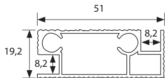
Sección perfil
