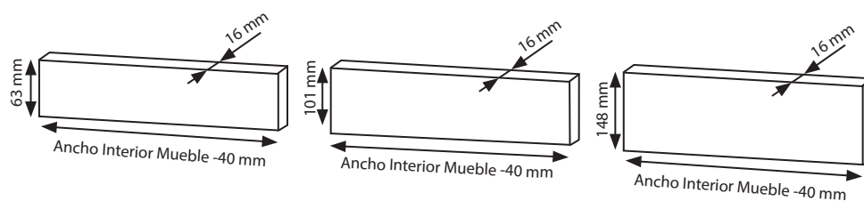
Trasera de Cajón
