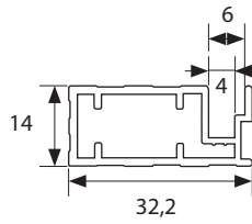
Sección perfil
