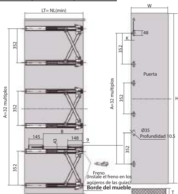
Medidas de instalación para 3 mecanismos
