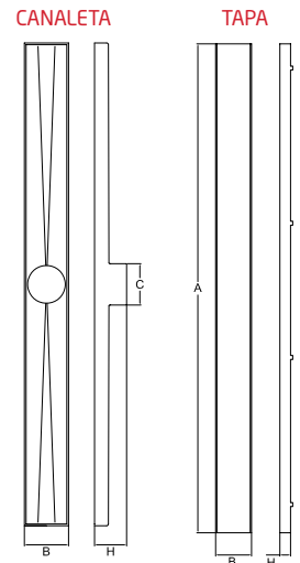
CUERPO SIFONADO
