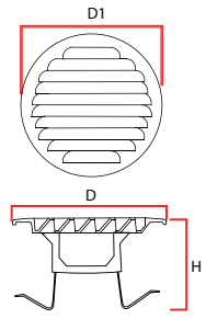
REJILLA DE COBRE REDONDA CON MUELLE
