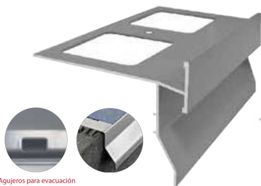
Agujeros para evacuación de agua debajo del azulejo
