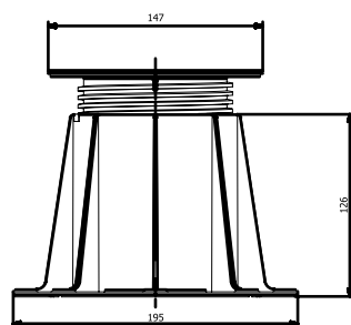
GB-K-A4 (133-225 mm)
