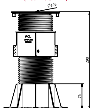
GB-K-A5 (189-293mm)
